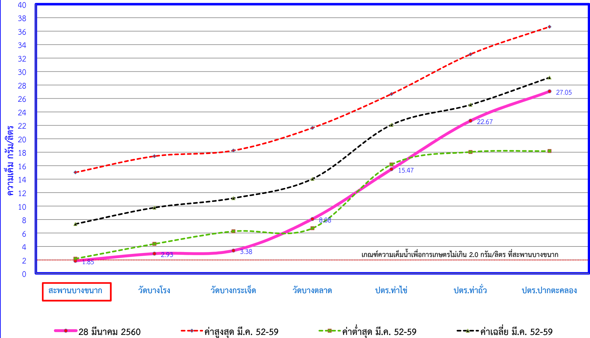
ค่าความเค็มในแม่น้ำบางปะกง วันที่ 28 มีนาคม พ.ศ. 2560
